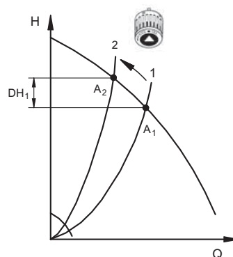
Abb. 16 Ungeregelte Pumpe
