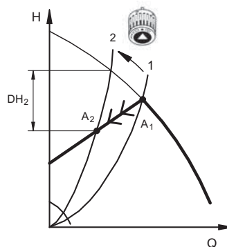
Abb. 17 Pumpe mit eingestellter Proportionaldruckregelung
