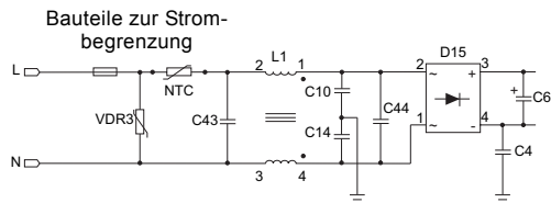
Abb. 42 NTC-Widerstand
